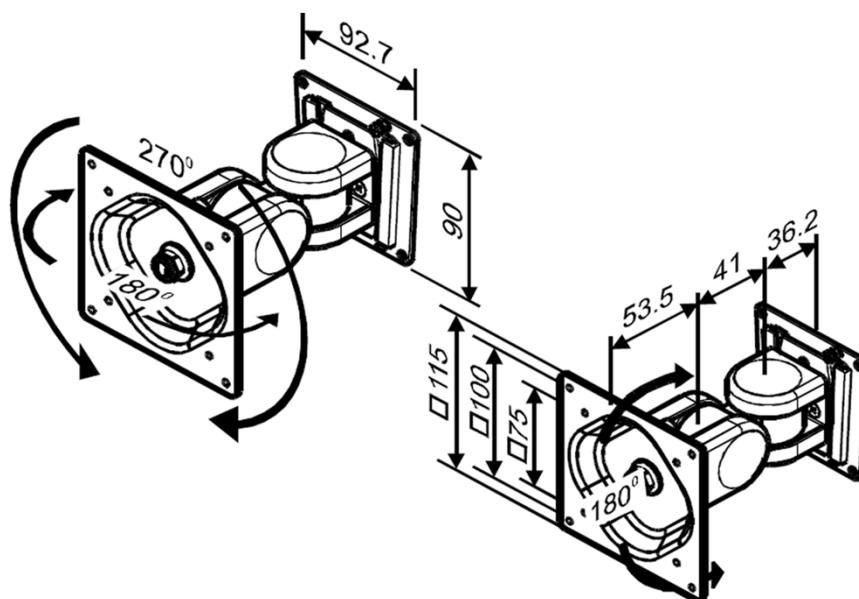
モニターを270° 回転可
